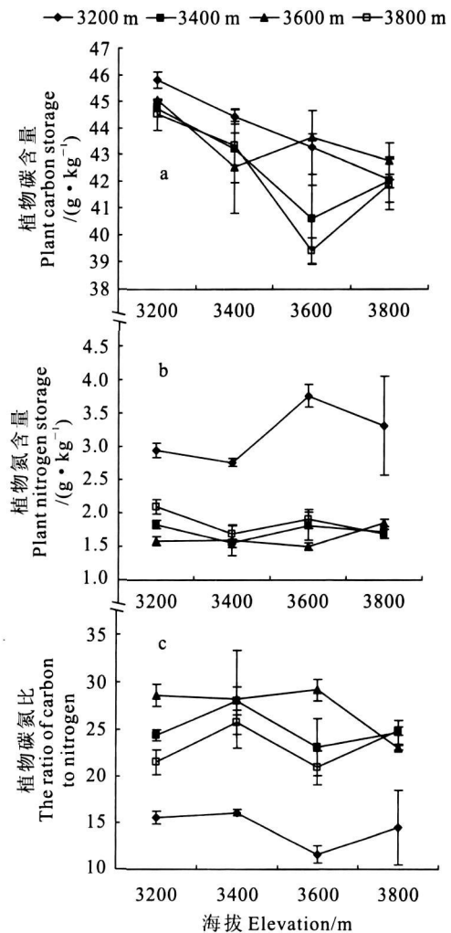
图1 植物群落的植物碳(a)、氮(b)及碳氮比(c)的变化特征 图例表示植物的原生地
